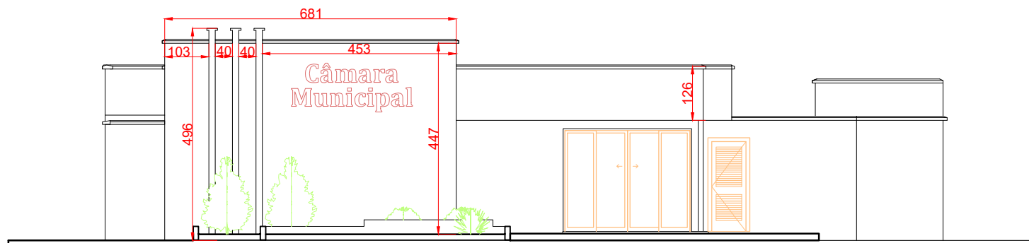
3 DETALHAMENTO - FACHADA ESC.: 1:125
