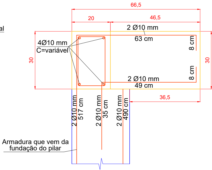
8 DETALHAMENTO - PILARES P1 A P8, VIGAS EM BALANÇO V1 A V8 E VIGAS PARALELAS À PAREDE V9 E V10 ESC.: 1:1
