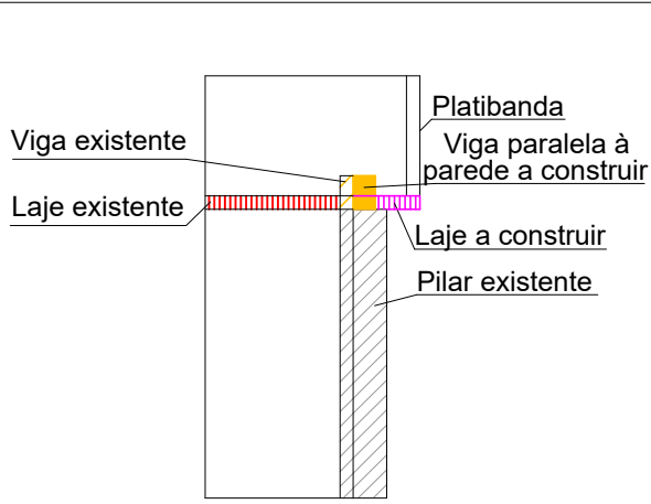
2 DETALHAMENTO 1 (DET 1) PILAR EXISTENTE ESC.: 1:75
