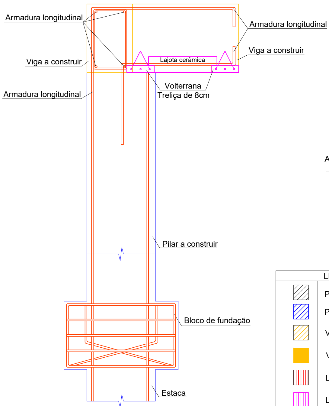
7 DETALHAMENTO - LIGAÇÃO DE PILAR A CONSTRUIR (P1 A P8), VIGAS E LAJE ESC.: 1:1
