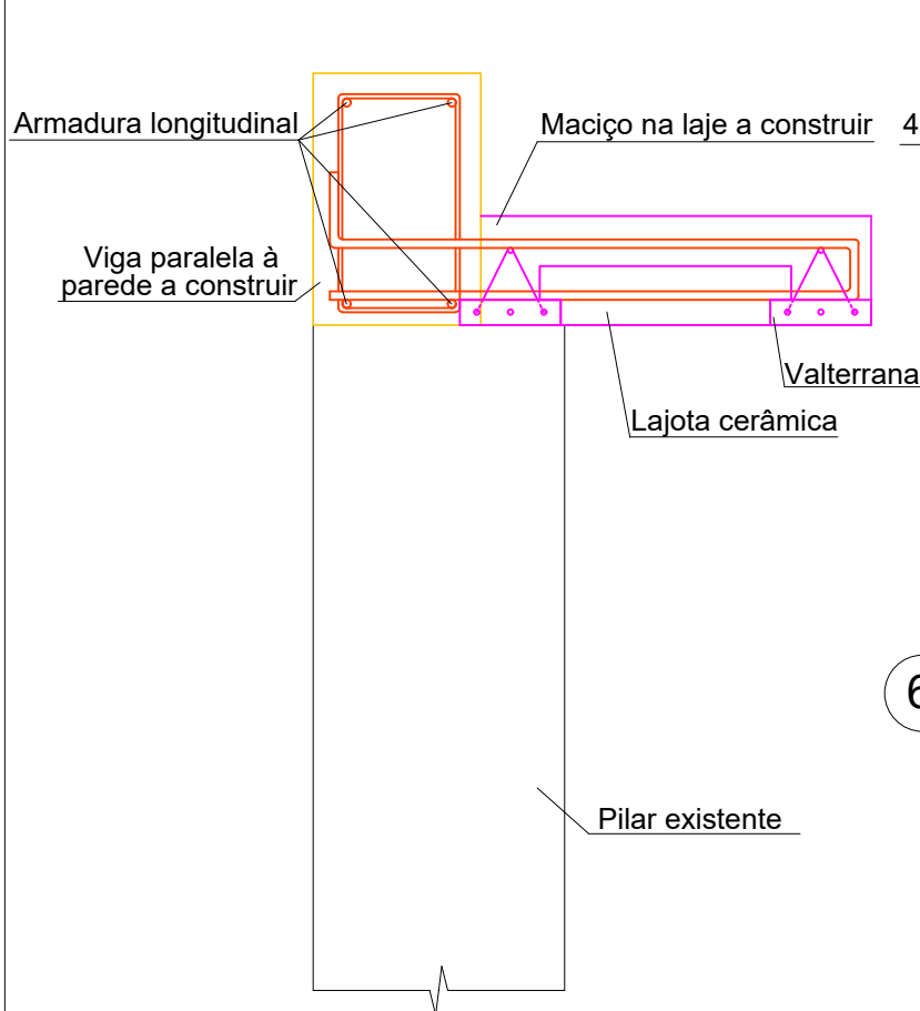
5 DETALHAMENTO - LIGAÇÃO DE PILAR EXISTENTE E VIGA E LAJE A CONSTRUIR ESC.: 1:1
