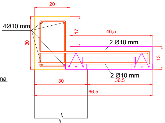
6 DETALHAMENTO DA ARMADURA - VIGAS V9 E V10 e MACIÇOS M1 A M5 ESC.: 1:1
