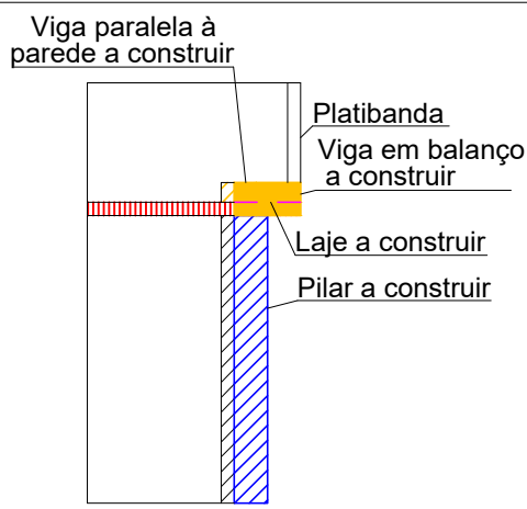
3 DETALHAMENTO 2 (DET 2) PILAR A CONSTRUIR ESC.: 1:75
