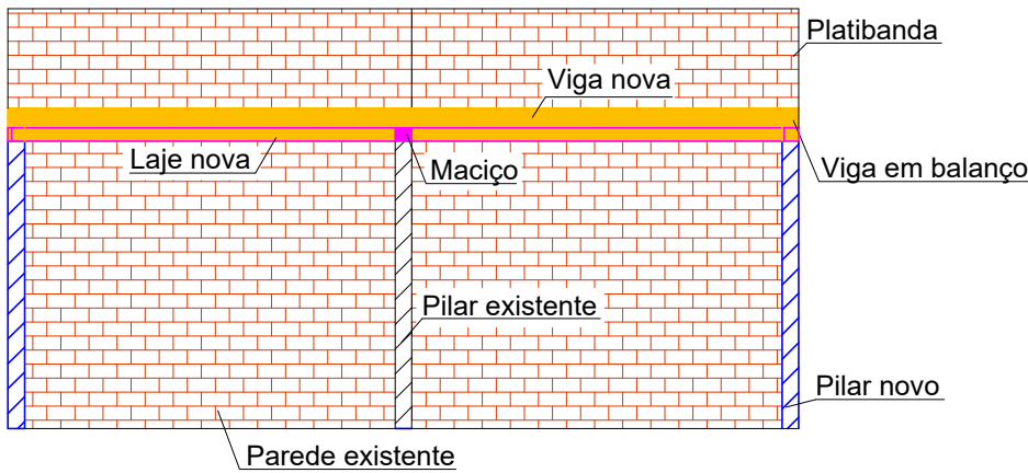
4 DETALHAMENTO GERAL ESC.: 1:75
